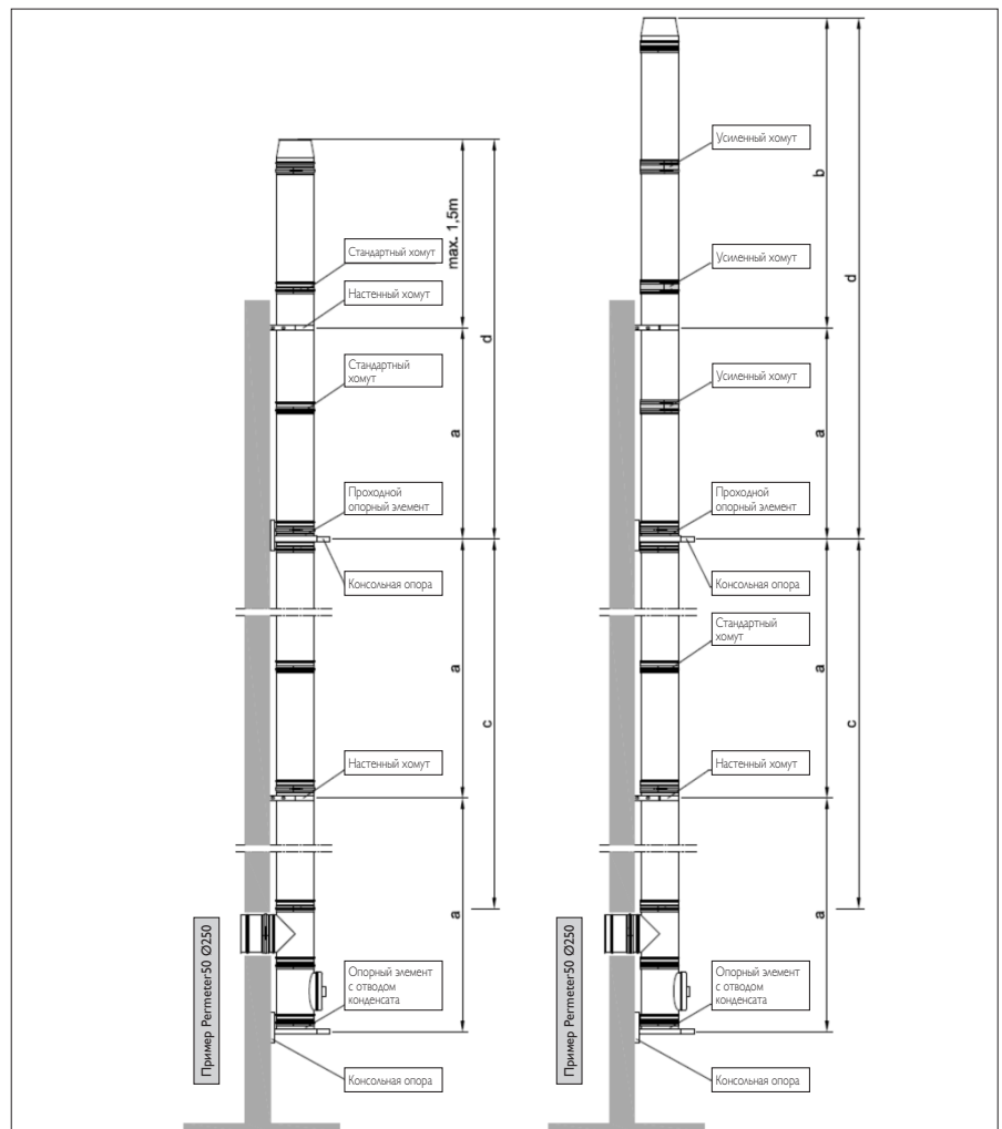
PERMETER50 Ø130-Ø250
